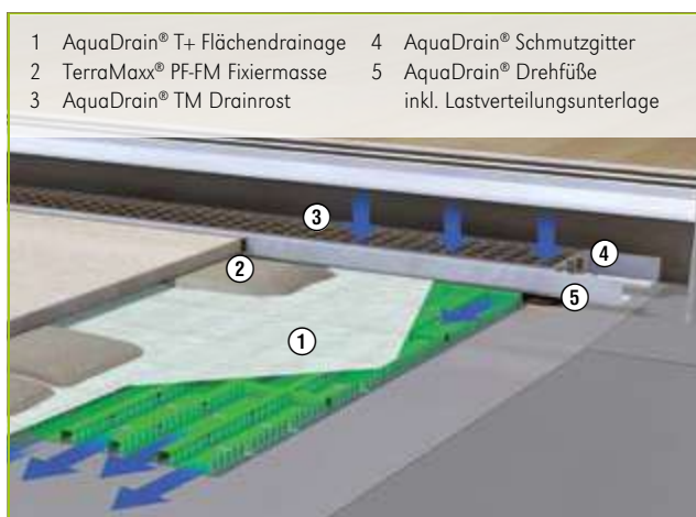
Extrem dünnere TerraMaxx ® PF Verlegung
