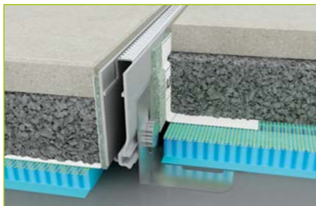
Aqua Drain® SR-U voor de lijndrainage
