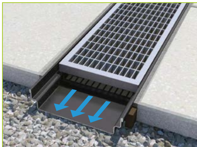
AquaDrain® KRU zonder sleuf als afvoerkanal
