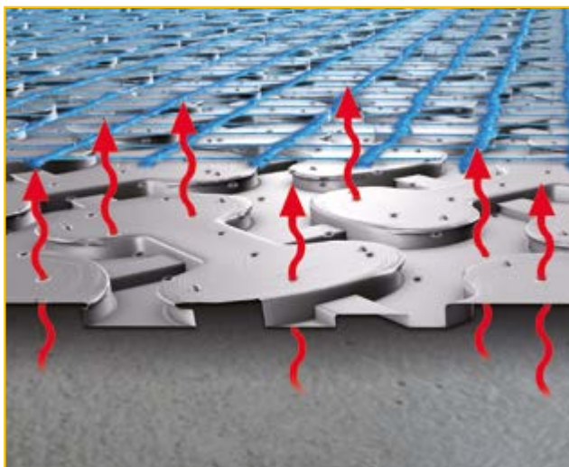
Restvocht in de ondergrond wordt gelijkmatig over het drainagesysteem verdeeld en kan door de perforaties in de mat via de voegen ontluften.
